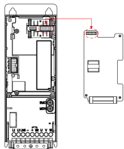
图2-2 PG扩展卡电气安装接口
