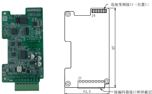
图1-1 PG外观
