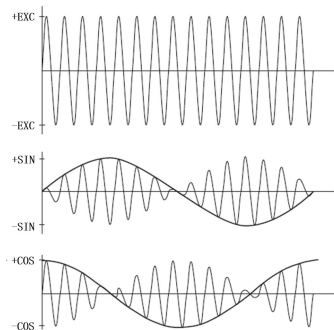
图1-3 旋变信号
