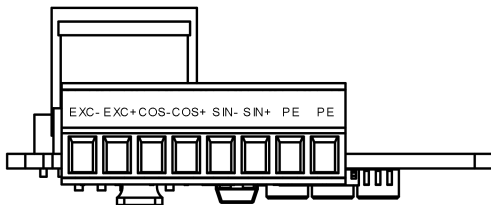
图1-2 端子丝印示意图
